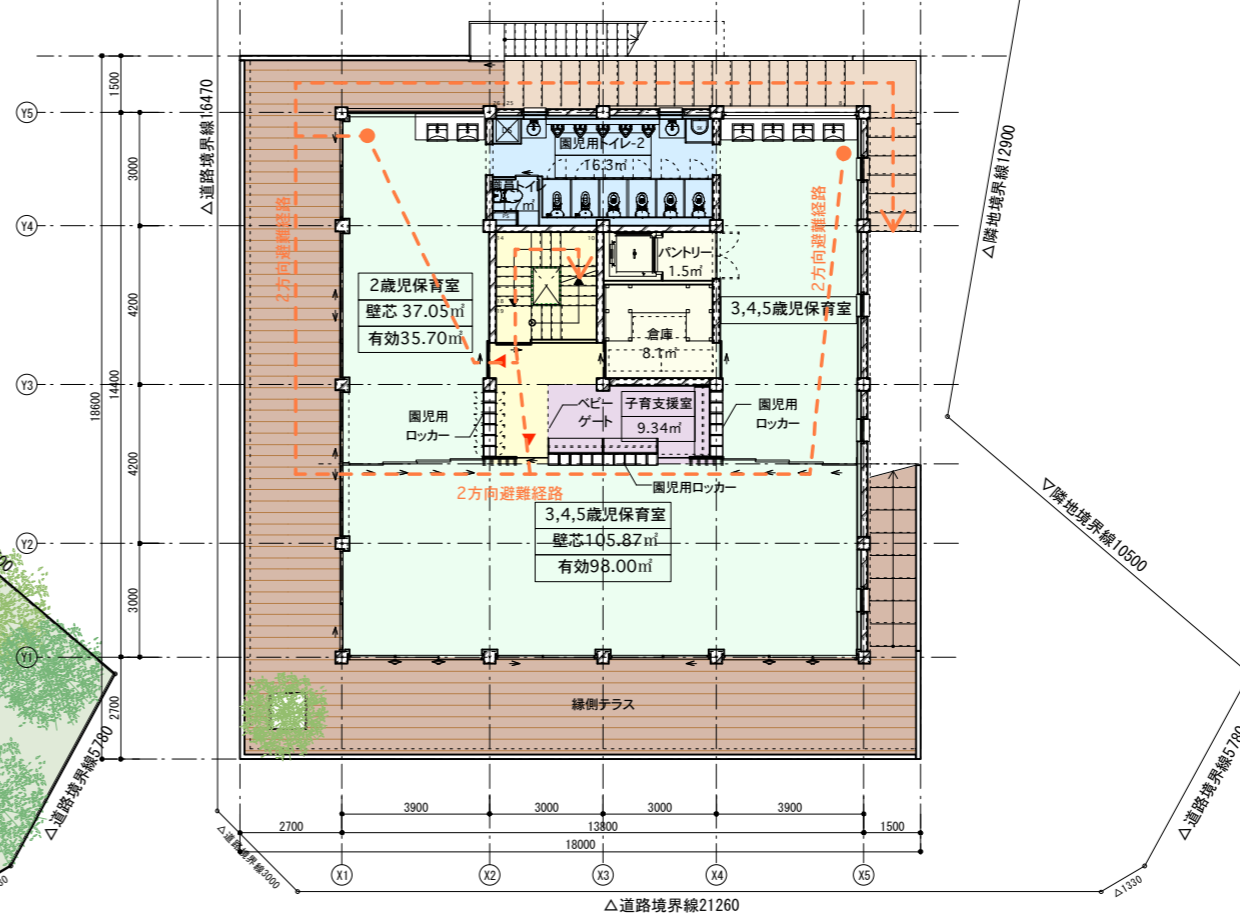
配置図兼1F平面図S=1:200
